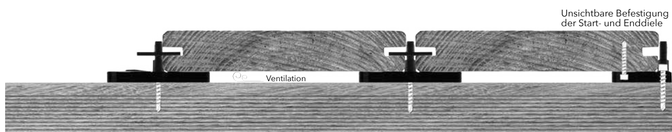
Empfohlenes Zubehör: 2 Stück UNIA1 Systemschrauben 4,2 x 17 mm pro Start- oder Endverbinder
